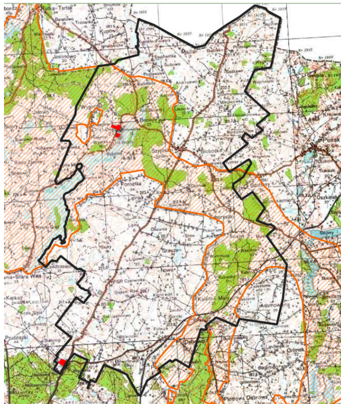
Granice uchwały intencyjnej na tle korytarzy ekologicznych wskazanych w PZPWP (GKPN-4A Puszcza Augustowska – Puszcza Romincka)
