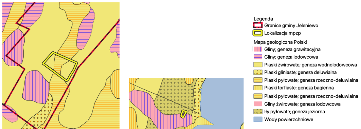
Ryc. 5 (z wykorzystaniem Szczegółowej mapy geologicznej Polski M. Bruj., P. Woźniak 1987) Szczegółowa mapa geologiczna PIG – brak arkuszy)
